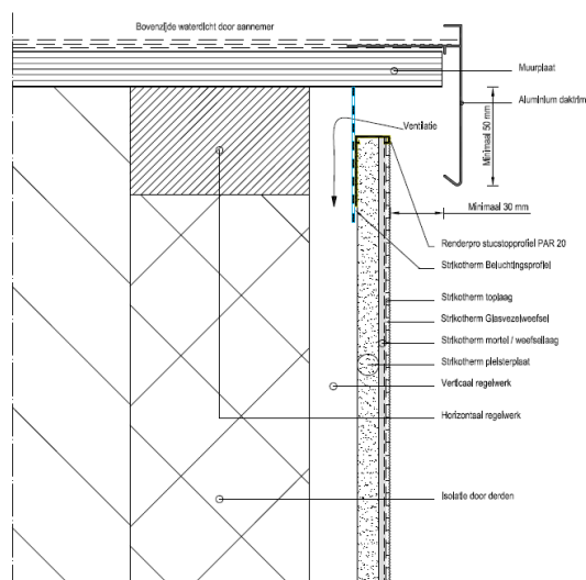
Aansluiting dakrand
